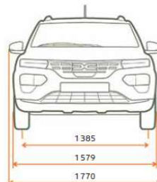
VEDERE FRONTALĂ
